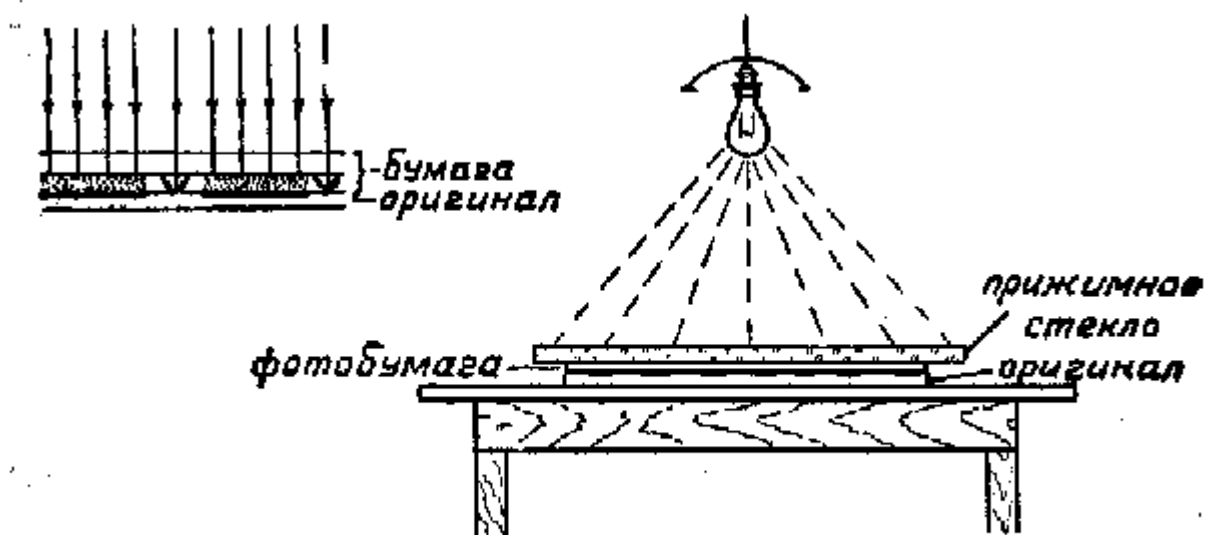
Рис. 25. Схема рефлексной печати
