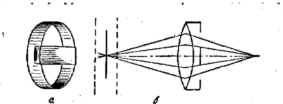
Рис. 17. Диафрагма-маска и принцип ее действия: а) общий вид диафрагмы, б) линии, параллельные перемычке диафрагмы, изобразятся резкими лишь в фокальной плоскости
